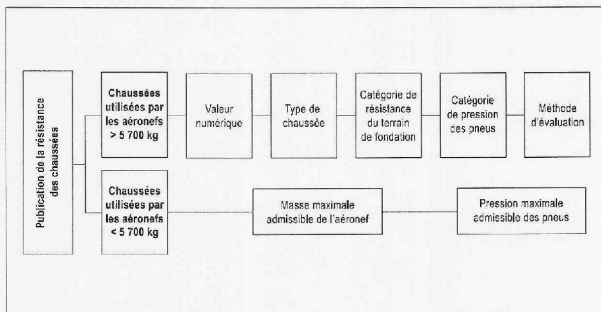
Figure 1. Détermination de la PCR
