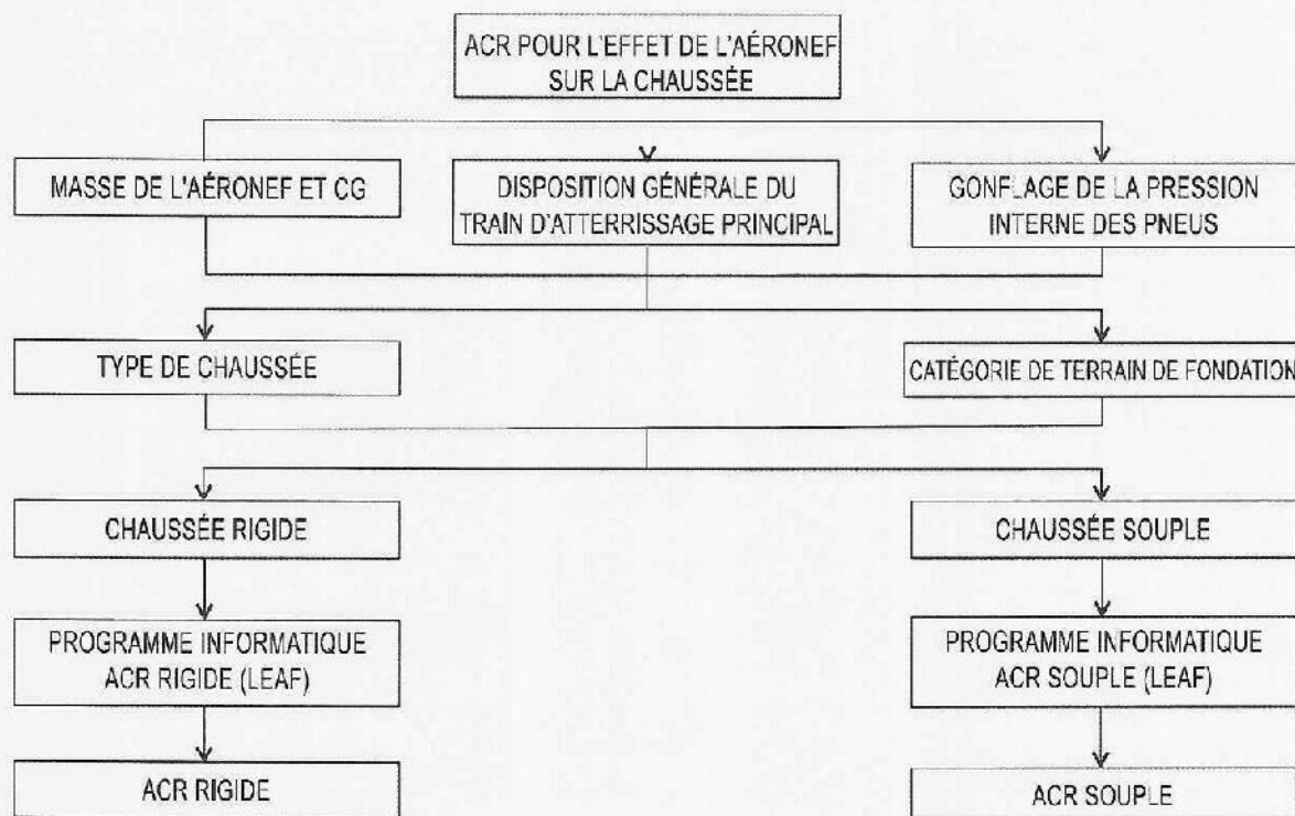
Figure 2. Calcul de l'ACR
