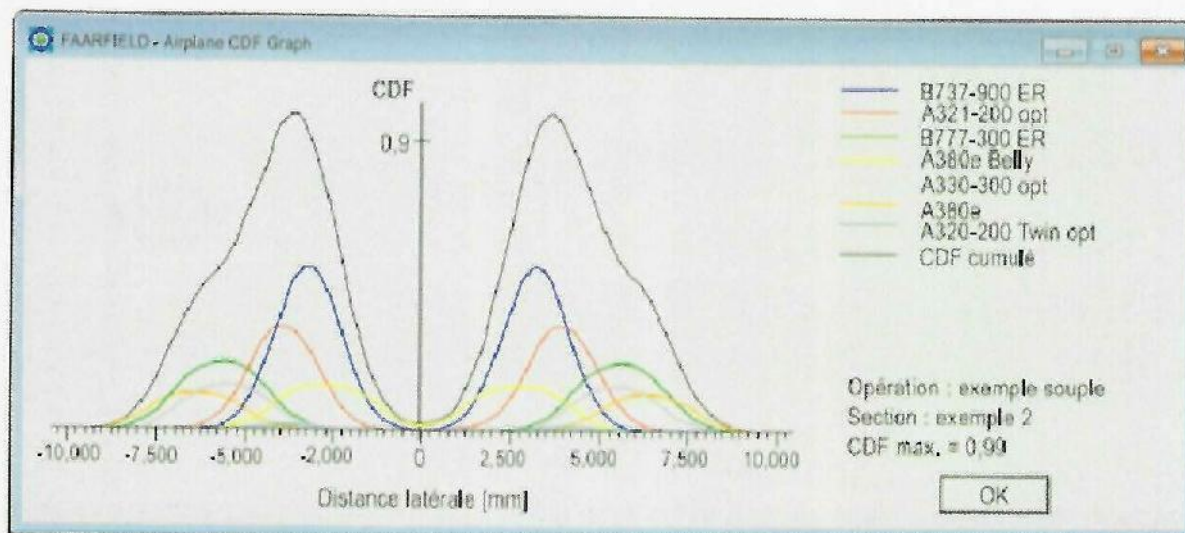
Figure 9. CDF de l'aéronef, CDF total et contribution de l'aéronef au CDF maximal
