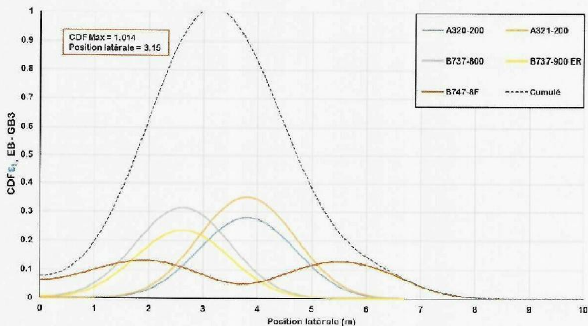
Figure 11. CDF de l'aéronef, CDF total et contribution de l'aéronef au CDF maximal
