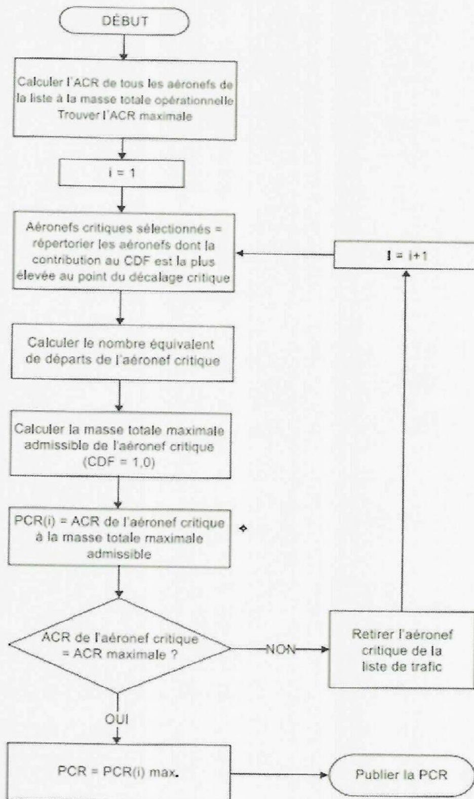
Figure 7. Logigramme d'évaluation technique de la PCR
