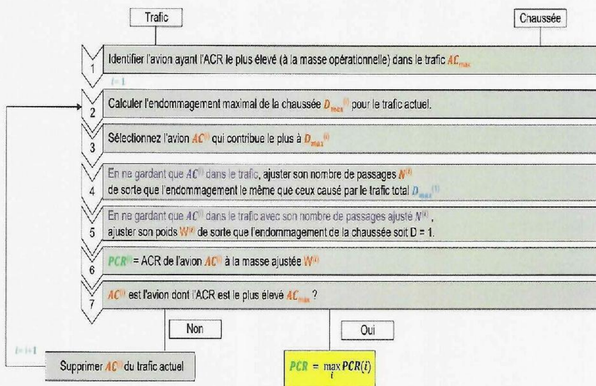
Figure 6. Représentation schématique de la procédure d'évaluation technique de la PCR d'une chaussée ( D_{max} représente le CDF_{max} )
