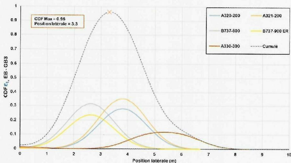
Figure 10. CDF de l'aéronef, CDF total et contribution de l'aéronef au CDF maximal
