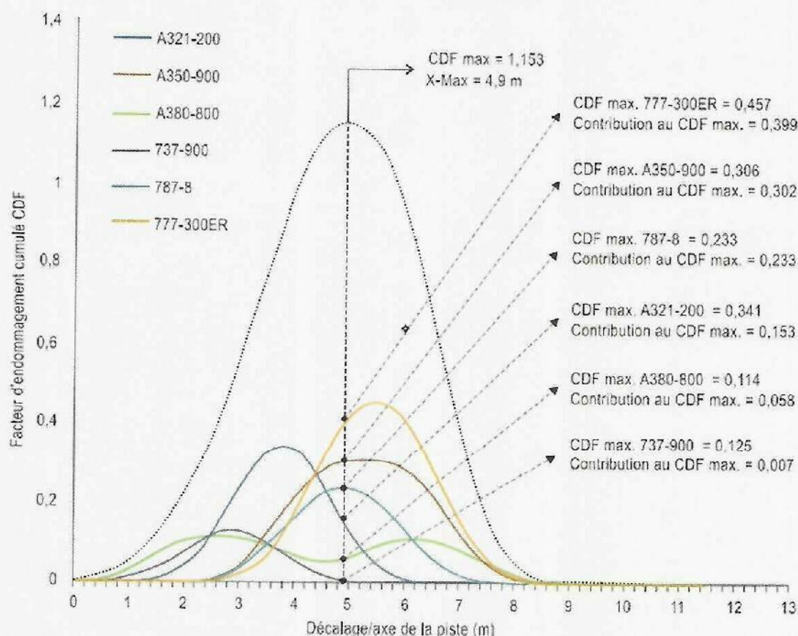
Figure 8. CDF de l'aéronef, CDF total et contribution de l'aéronef au CDF maximal
